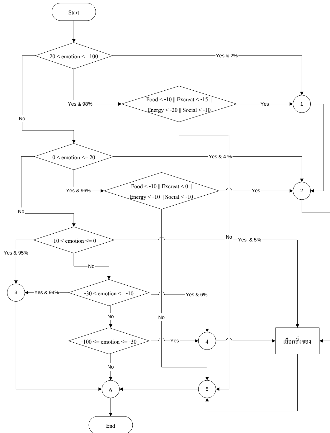
รูปที่ 3.5 แสดง Flow Chart แสดงการตัดสินใจเลือกหรือไม่เลือกสิ่งของของ NPC
